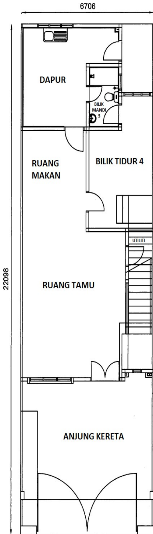
PELAN LANTAI TINGKAT BAWAH RUMAH TERES 2 TINGKAT - JENIS C
