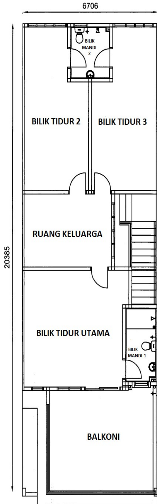
PELAN LANTAI TINGKAT SATU RUMAH TERES 2 TINGKAT - JENIS C
