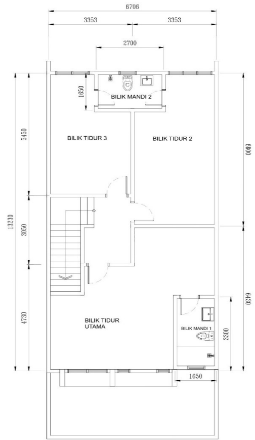
PELAN LANTAI TINGKAT 1
