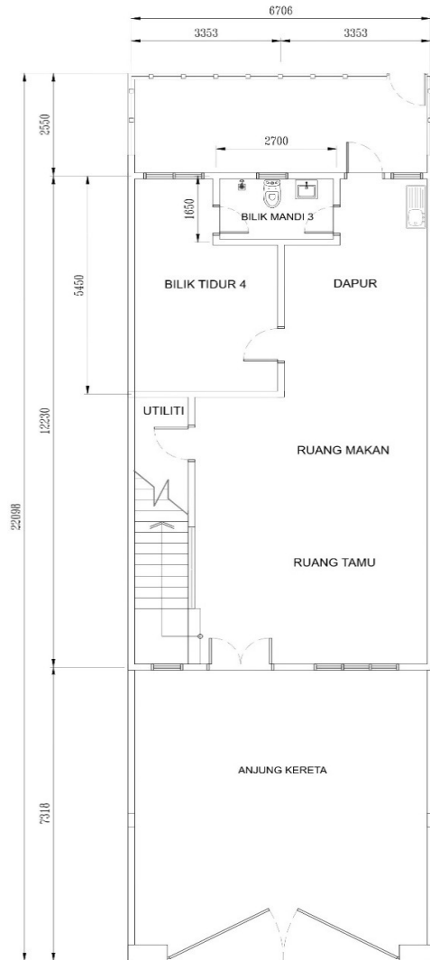
PELAN LANTAI TINGKAT BAWAH
