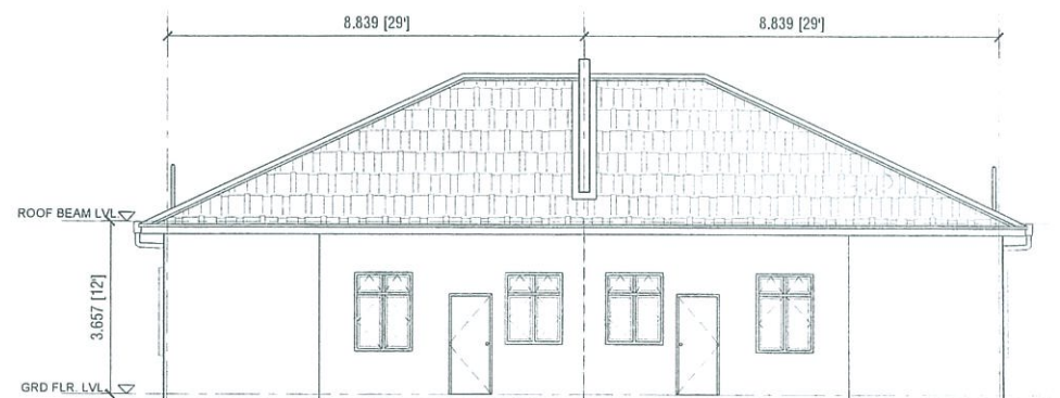
PANDANGAN BELAKANG (JENIS B)
