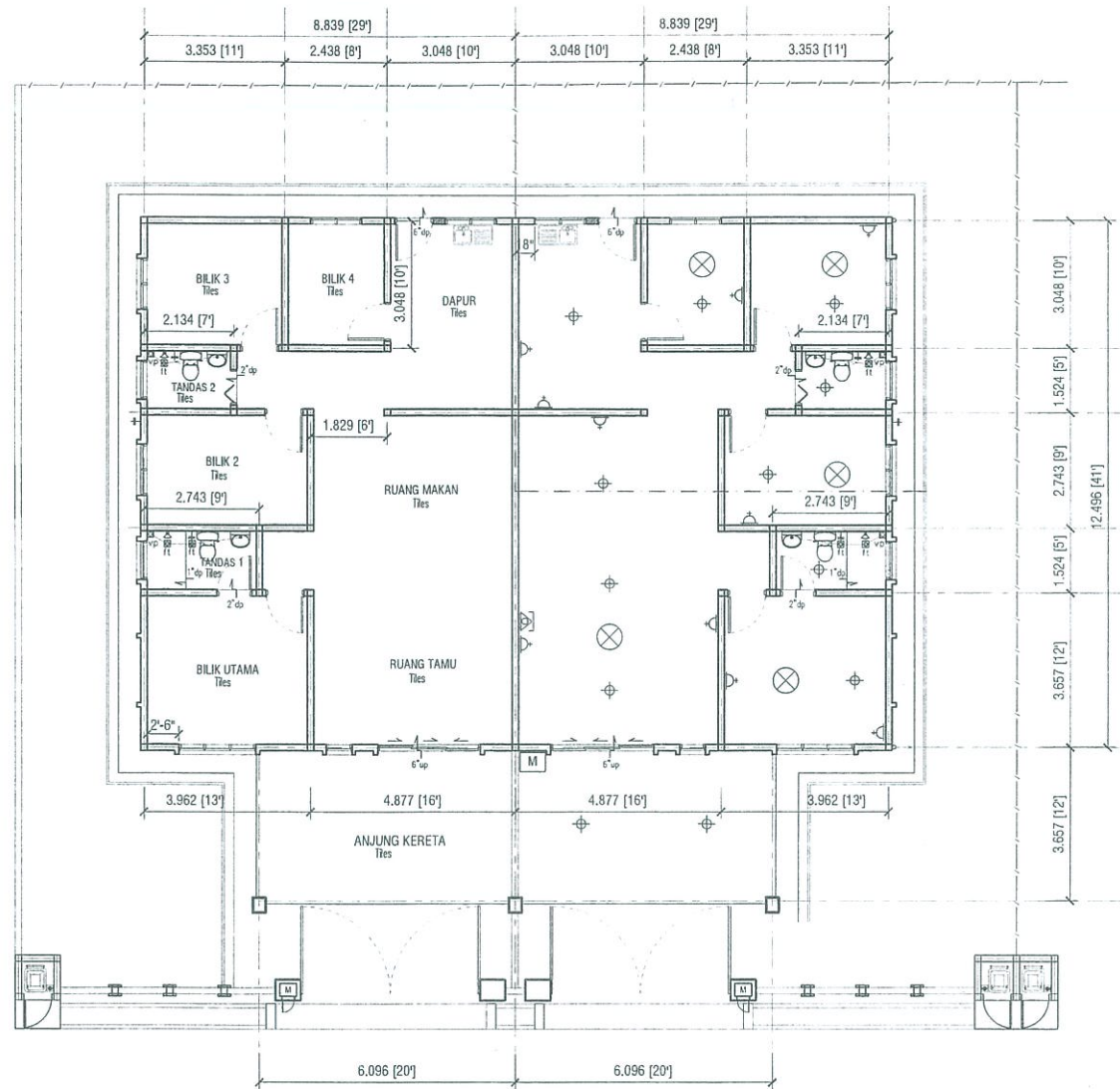
PELAN LANTAI (JENIS B)
