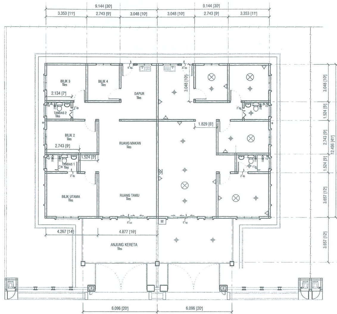
PELAN LANTAI (JENIS A) RUMAH BERBANDUNG SATU TINGKAT (SINGLE STOREY)
