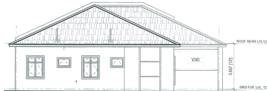
PANDANGAN SISI (JENIS B)
