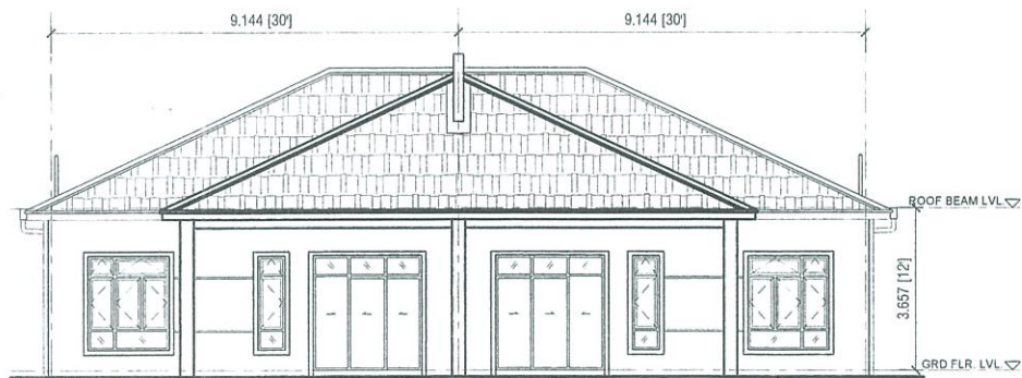
PANDANGA HADAPAN ( JENIS A )
