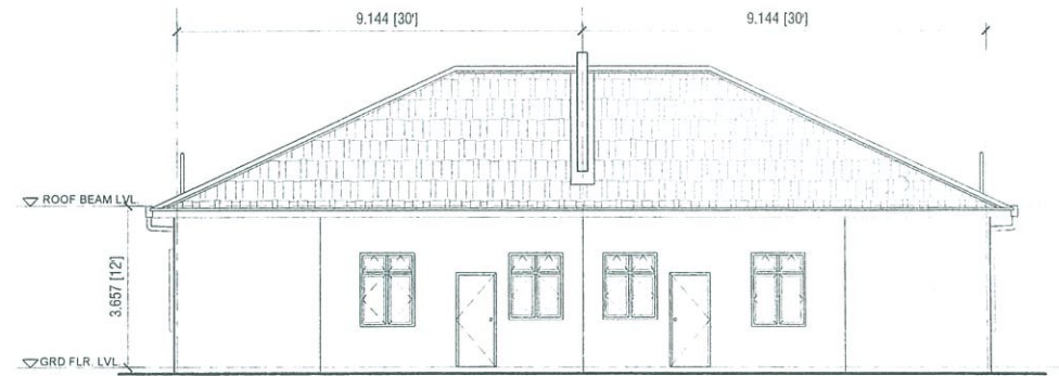
PANDANGAN BELAKANG ( JENIS A )
