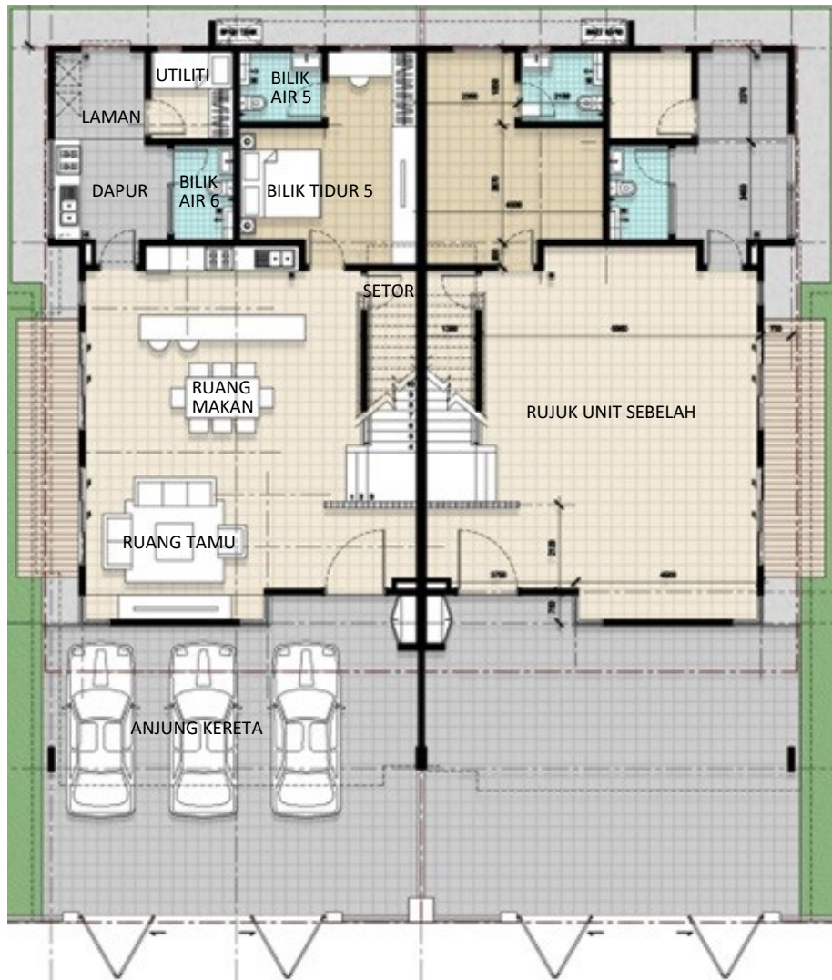
Pelan Bawah
