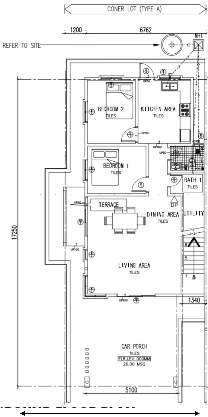
TINGKAT BAWAH
