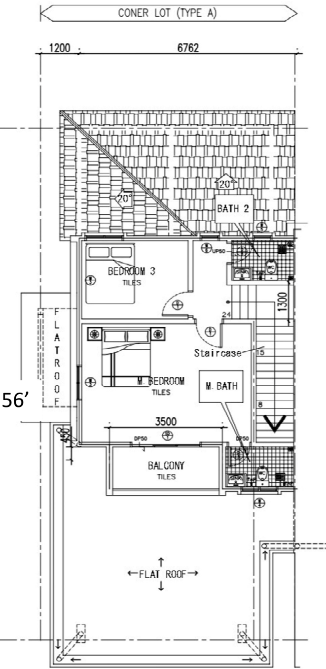
TINGKAT ATAS
