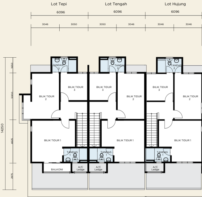
TINGKAT 1
