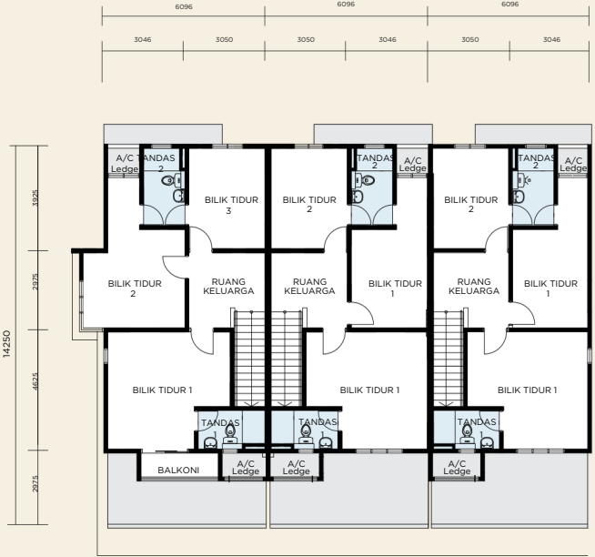
TINGKAT 1
