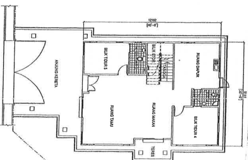
PELAN LANTAI BAWAH
