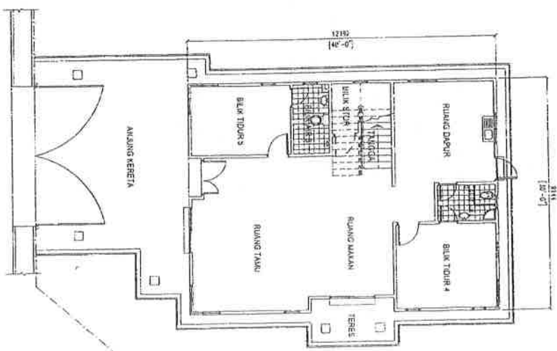
PELAN LANTAI BAWAH
