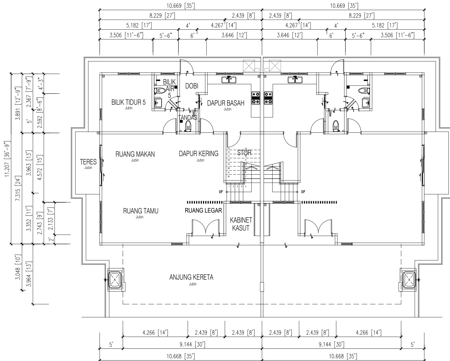
PELAN TINGKAT BAWAH
