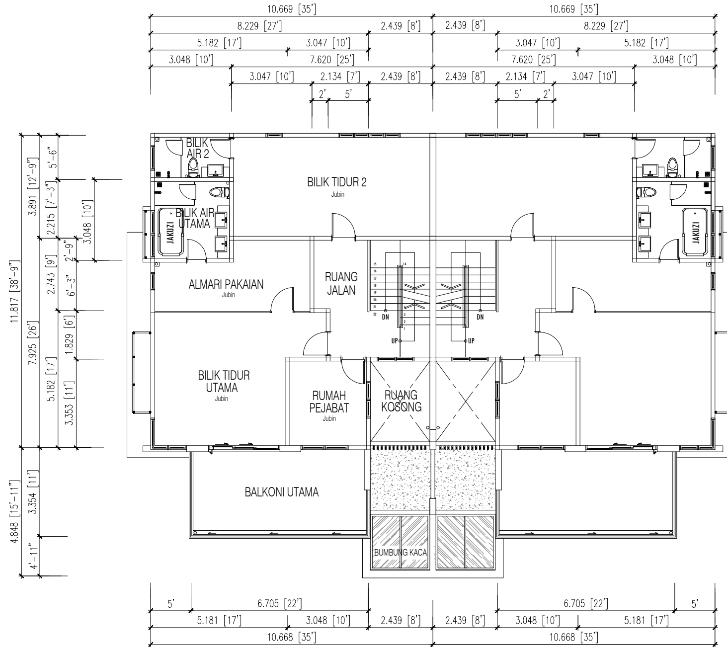
PELAN TINGKAT SATU
