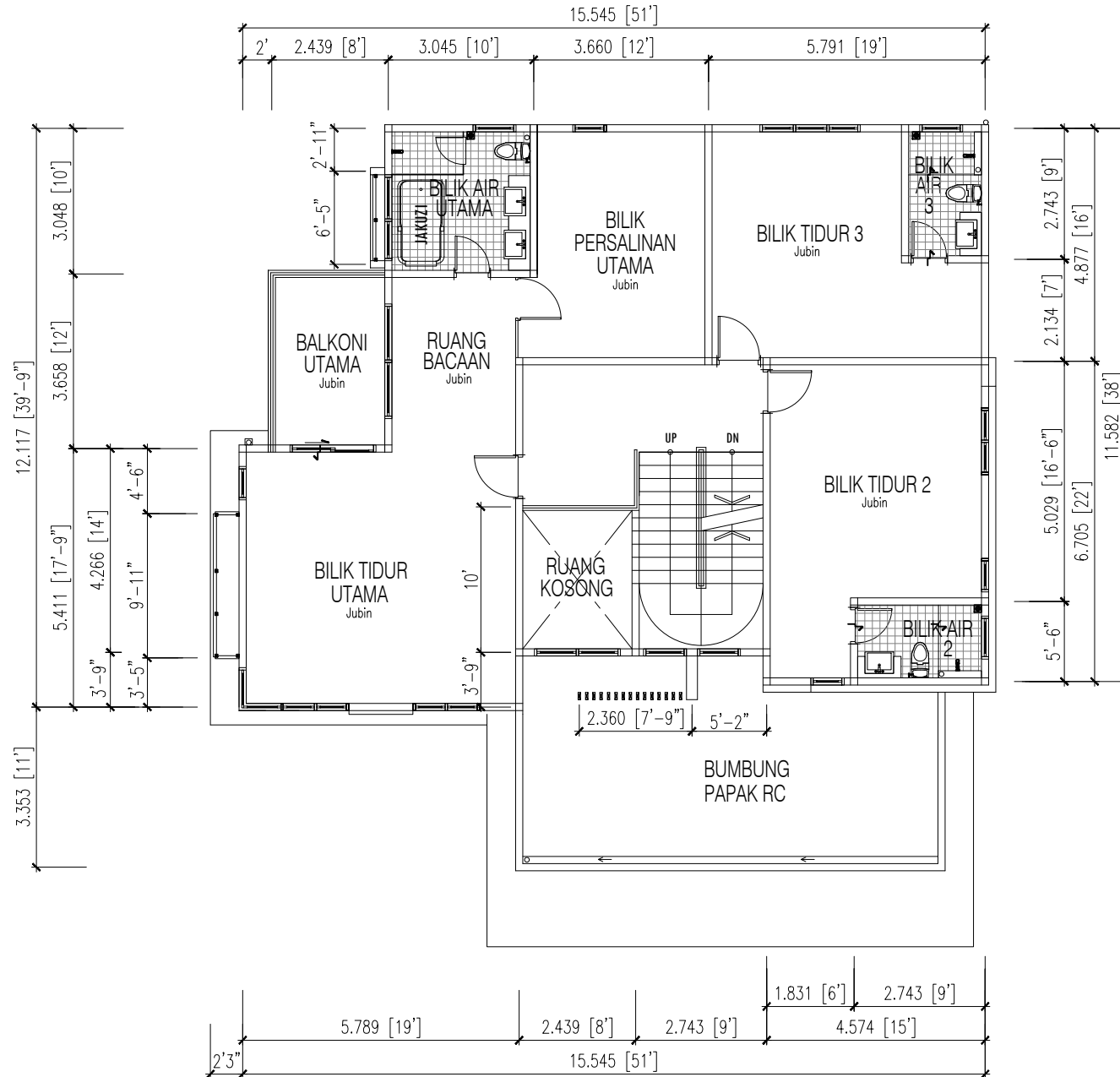
PELAN TINGKAT SATU
