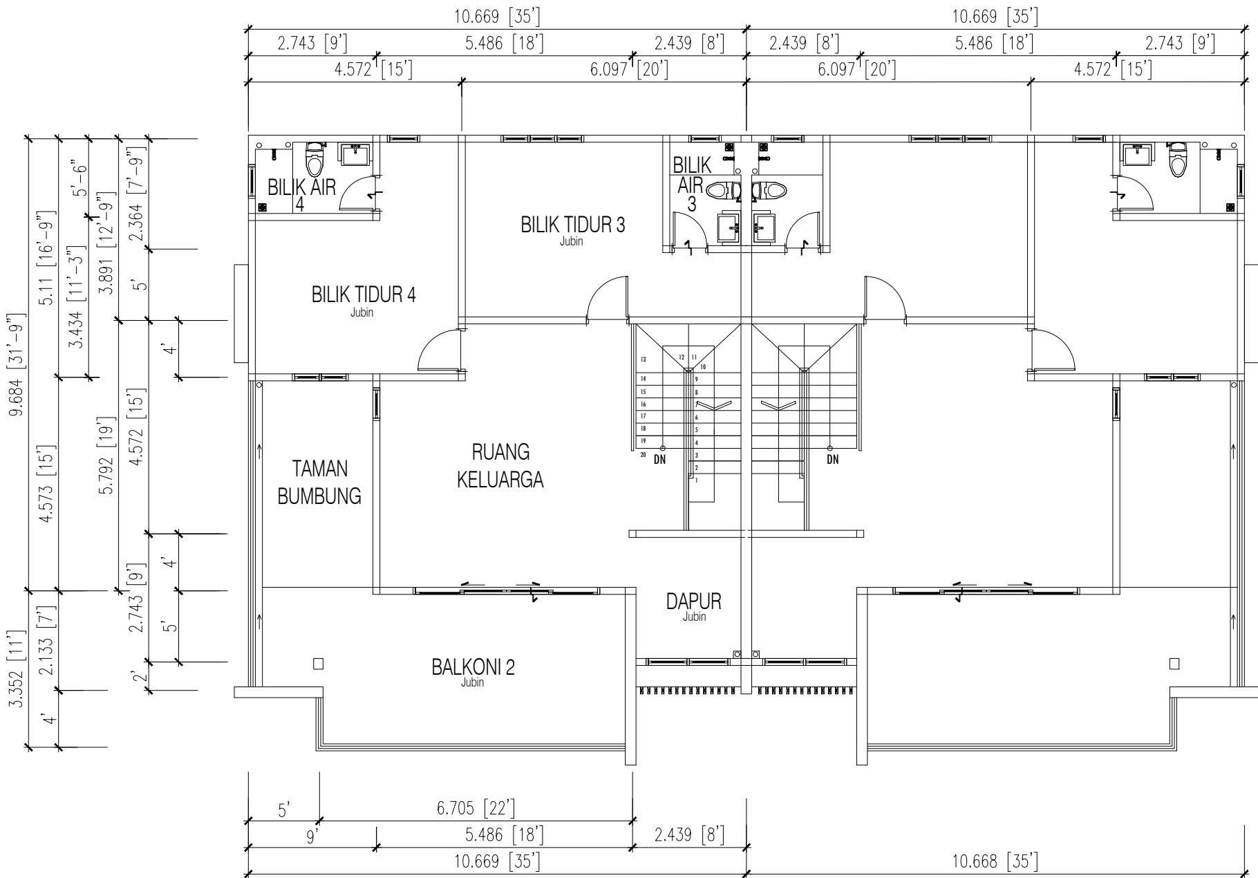
PELAN TINGKAT DUA
