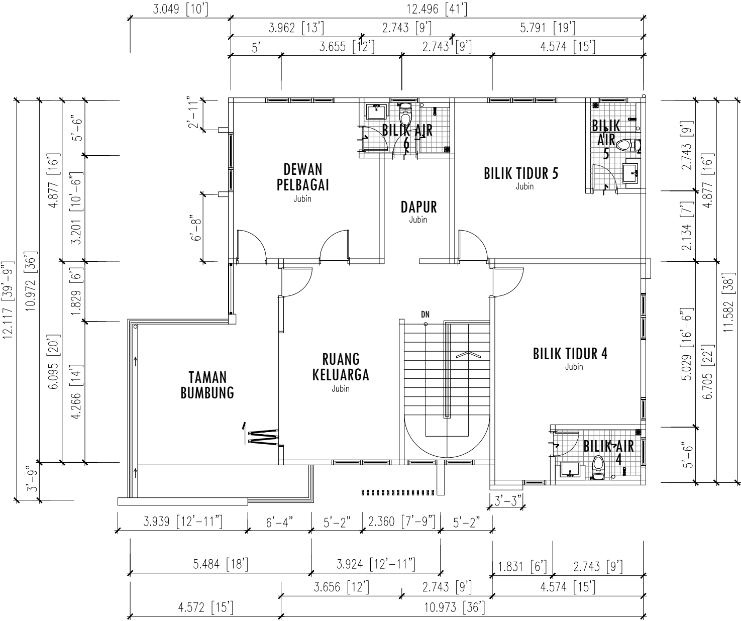
PELAN TINGKAT DUA
