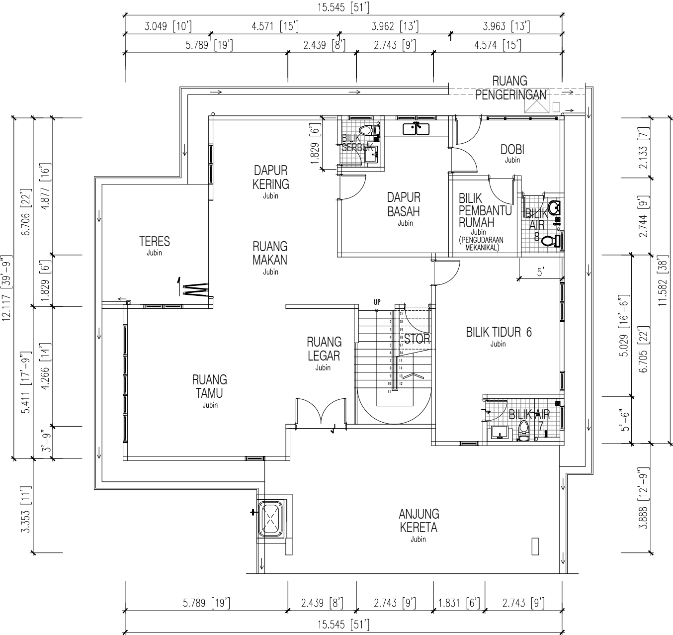
PELAN TINGKAT BAWAH
