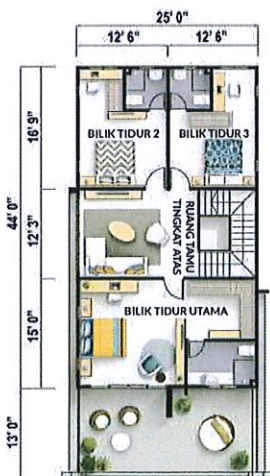
PELAN LANTAI TINGKAT ATAS DAN BAWAH
