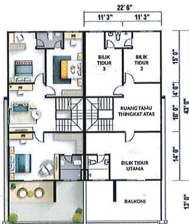
PELAN LANTAI TINGKAT ATAS DAN BAWAH
