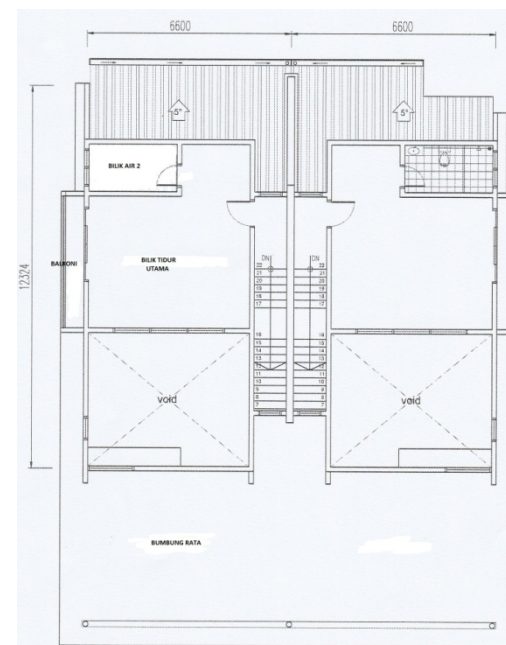
PELAN LANTAI ATAS
