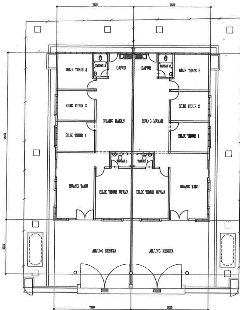
PELAN LANTAI RUMAH BERKEMBAR 1 TINGKAT
