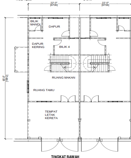
TINGKAT BAWAH
