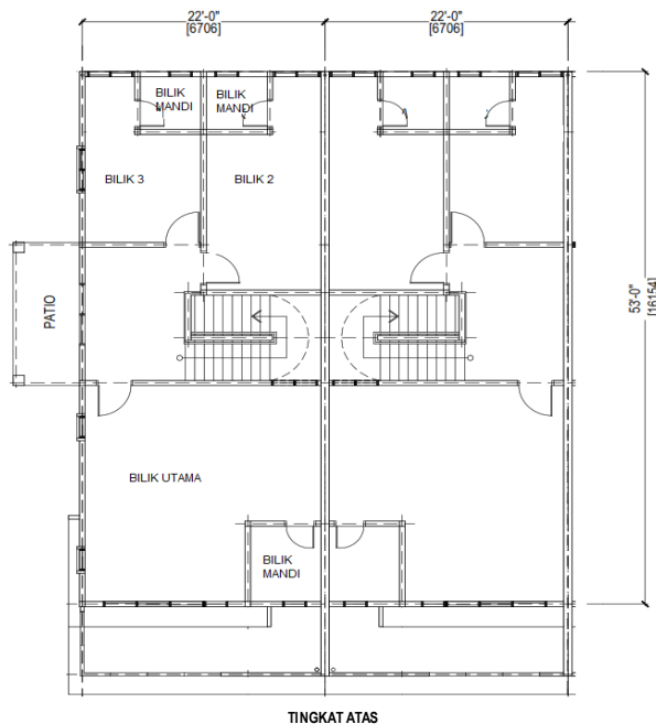
TINGKAT ATAS
