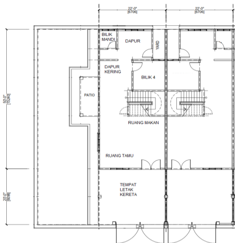
TINGKAT BAWAH
