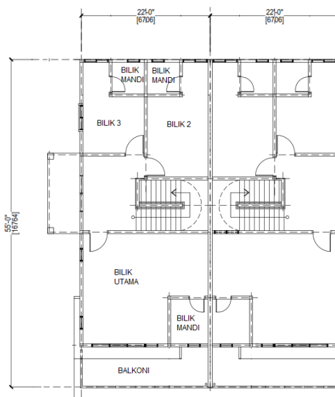
TINGKAT ATAS
