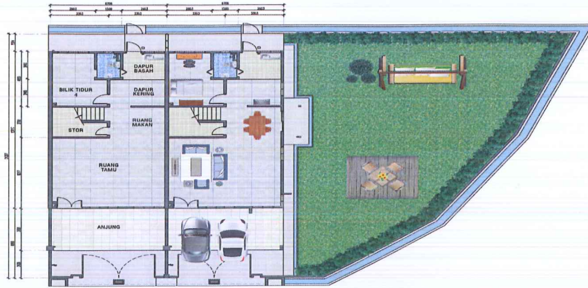
RUMAH TERES 2 TINGKAT (JENIS AMETHYST)
