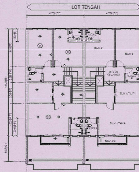
PELAN LANTAI TIPIKAL TINGKAT SATU
