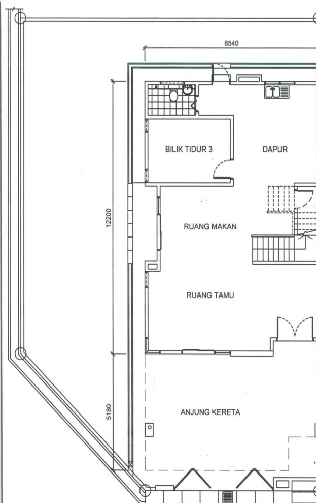
Pelan Lantai bawah
