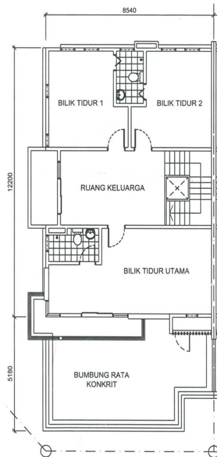
Pelan Lantai Atas
