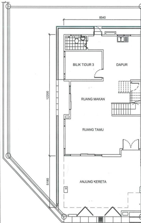
Pelantai bawah
