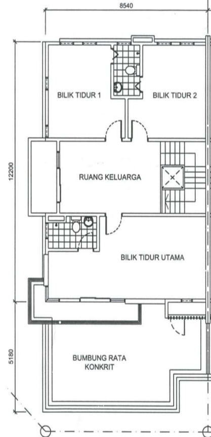
Pelantai Atas
