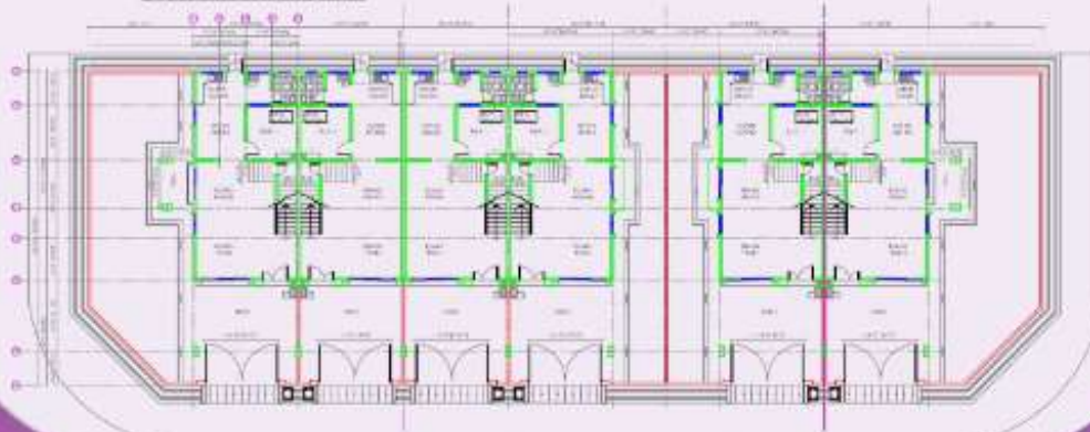
PELAN LANTAI TINGKAT BAWAH
