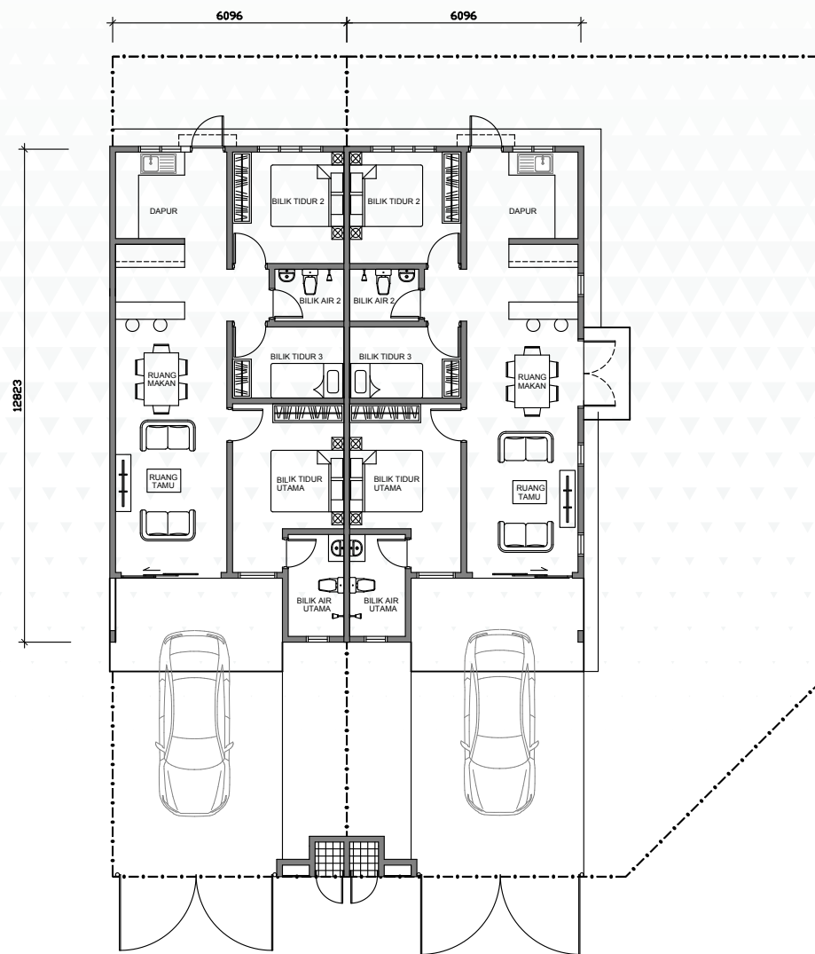
PELAN LANTAI UNIT TENGAH
