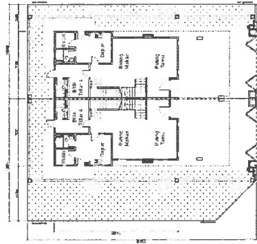
Tingkat Bawah
