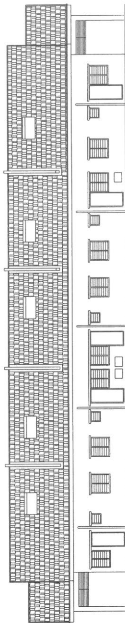
PANDANGAN BELAKANG
