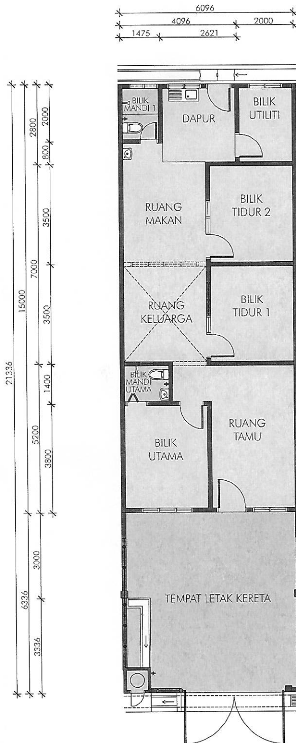
Rumah Teres 1 Tingkat (Luas binaan 1,178 k.p.s)
