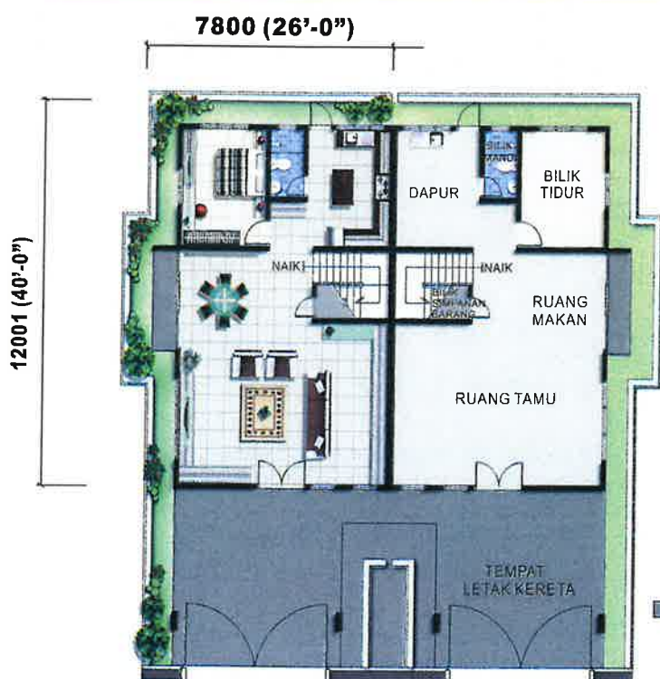
RUMAH BERKEMBAR 2 TINGKAT PLAN LANTAI TINGKAT BAWAH (26' X 40')
