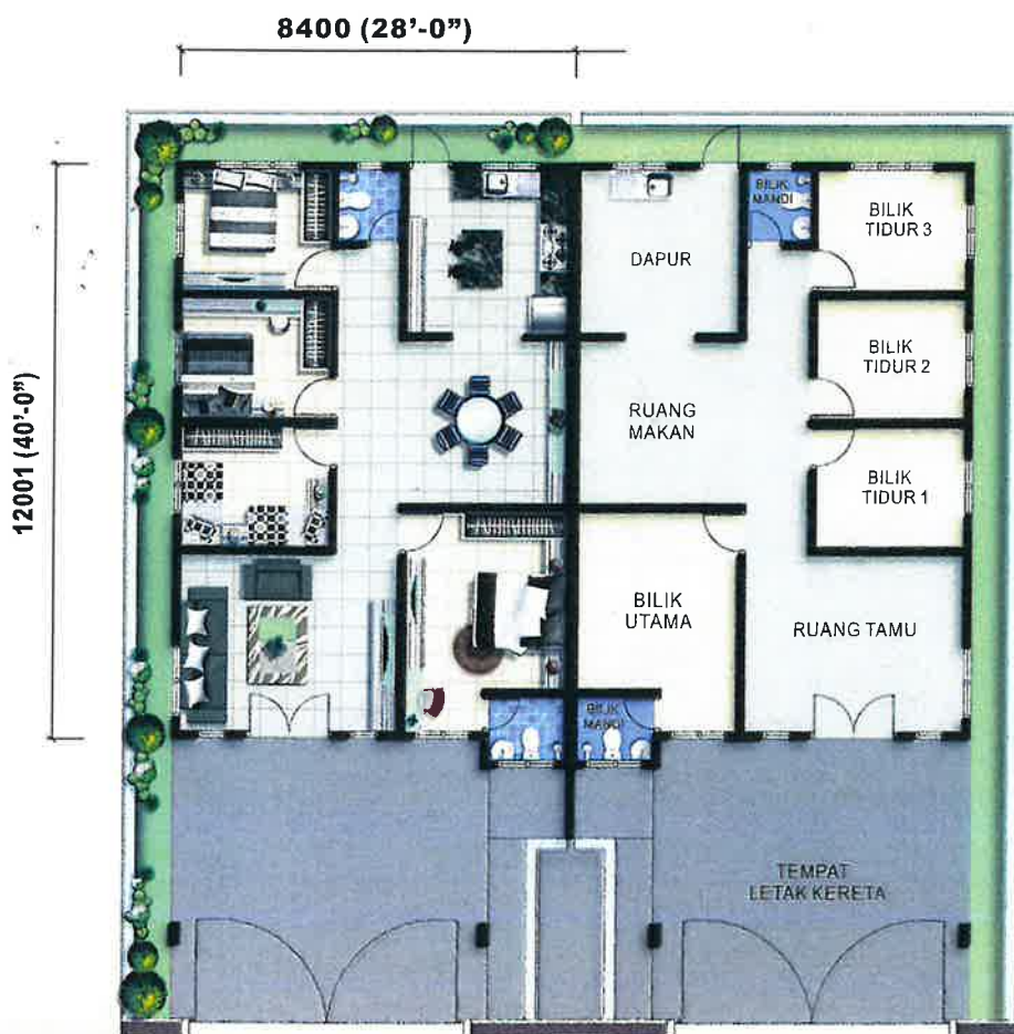
RUMAH BERKEMBAR 1 TINGKAT PELAN LANTAI (28' X 40')
