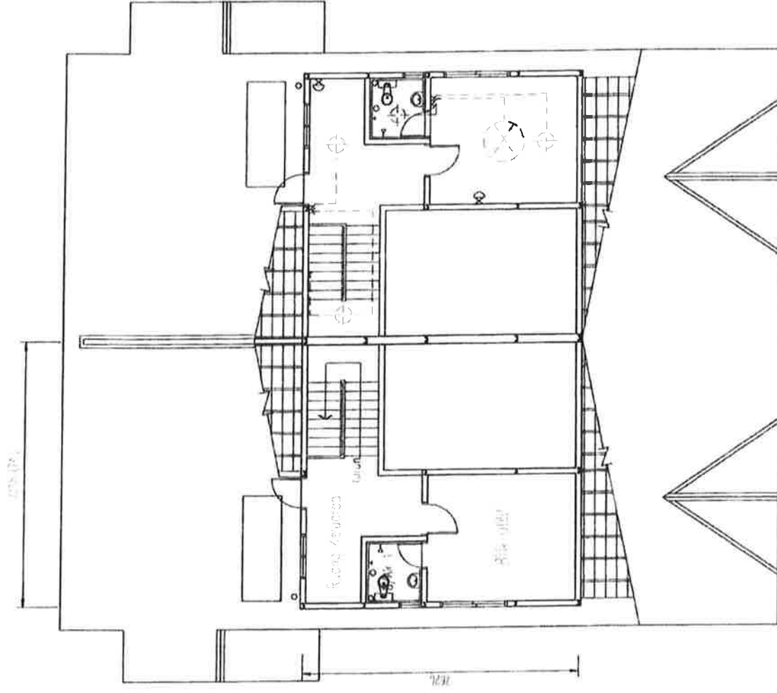
PELAN LANTAI MEZANIN
