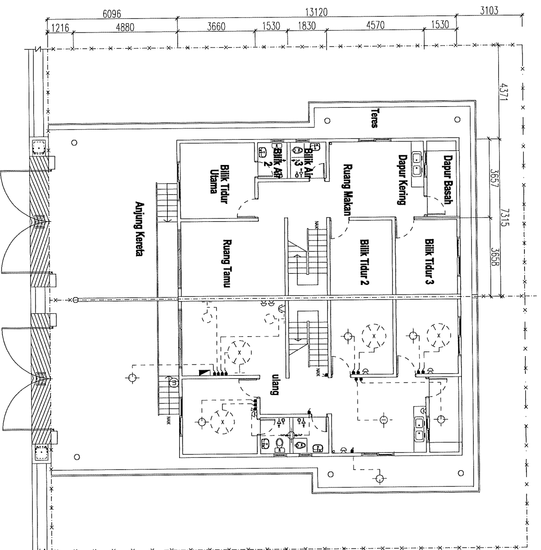
PELAN LANTAI
