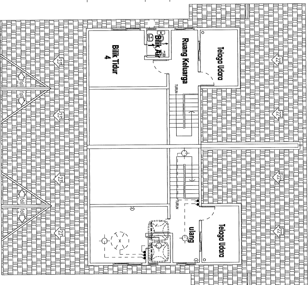
PELAN LANTAI MEZANIN
