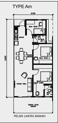
Pelan Lantai Am UNIT TENGAH
