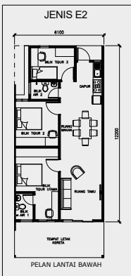
Pelan Lantai E2 UNIT SUDUT
