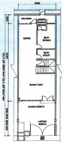
PELAN LANTAI
