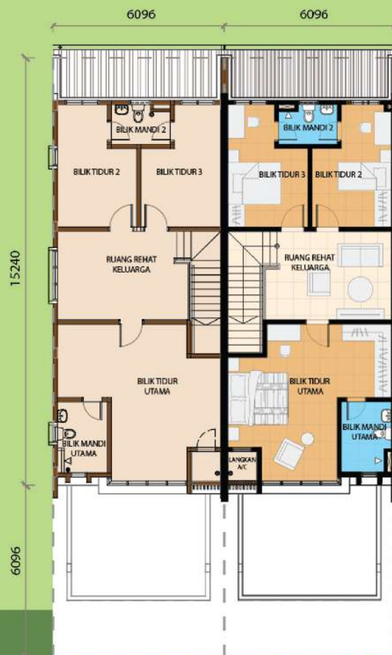
Pelan Tingkat Satu
