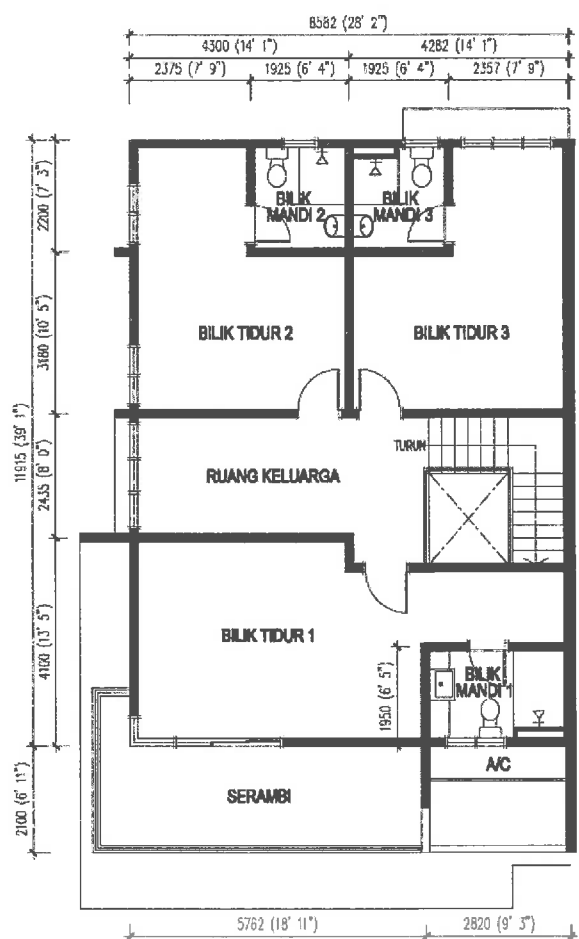
PELAN TINGKAT SATU
