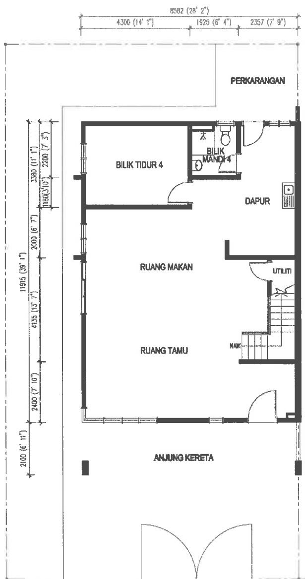
PELAN TINGKAT BAWAH
