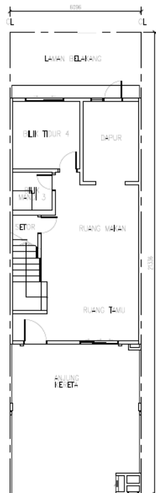
PELAN LANTAI BAWAH
