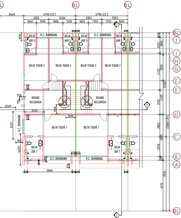
PLAN TINGKAT 1
