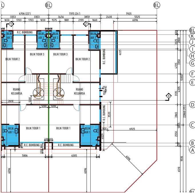
PLAN TINGKAT 1
