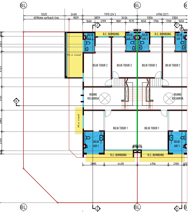
PLAN TINGKAT 1
