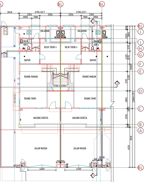
PLAN TINGKAT BAWAH
