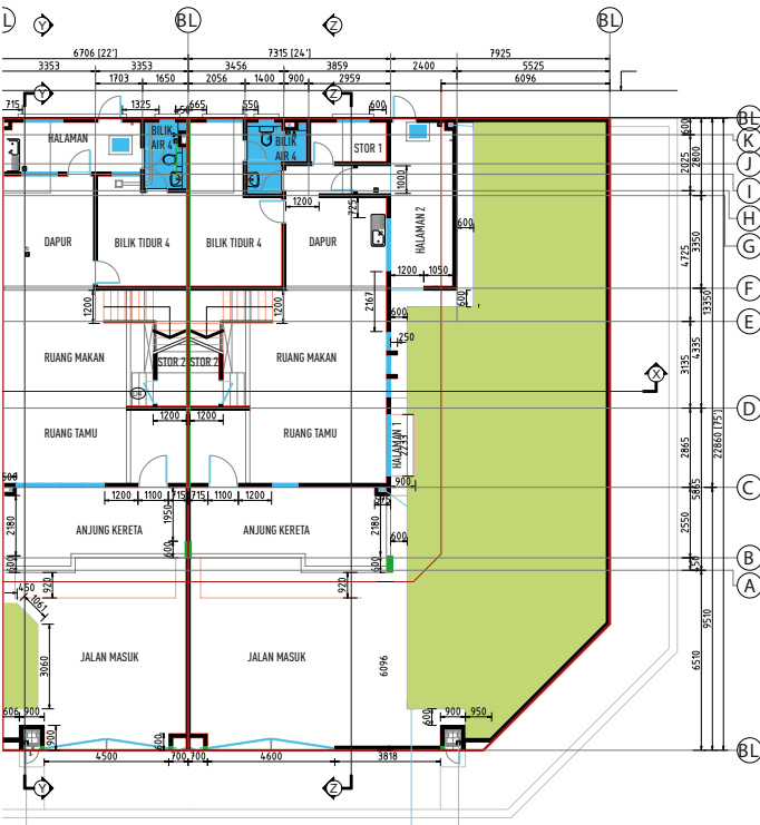
PLAN TINGKAT BAWAH
