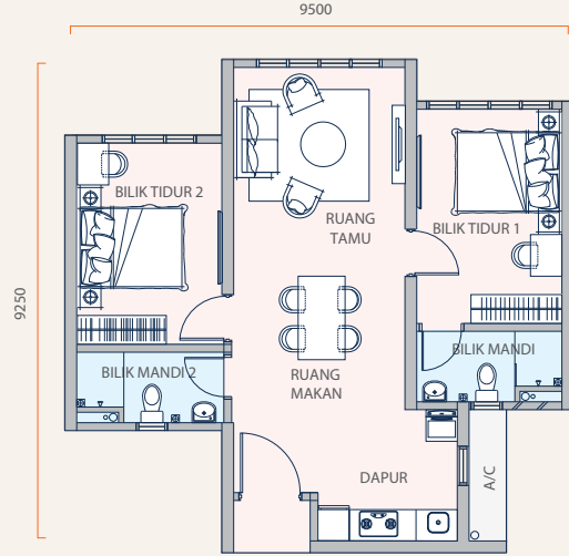
JENIS B 2 BILIK TIDUR 2 BILIK MANDI 763 KPS.
