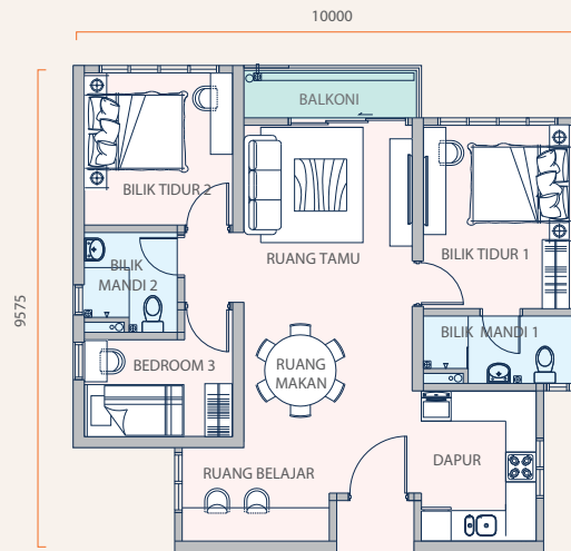
TYPE C2 3 BILIK TIDUR 2 BILIK MANDI 924 KPS.
