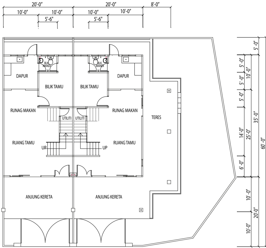
PELAN TINGKAT BAWAH
