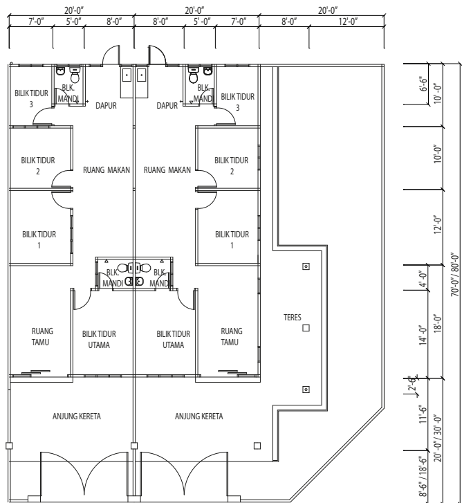
PELAN LANTAI_Jenis A
