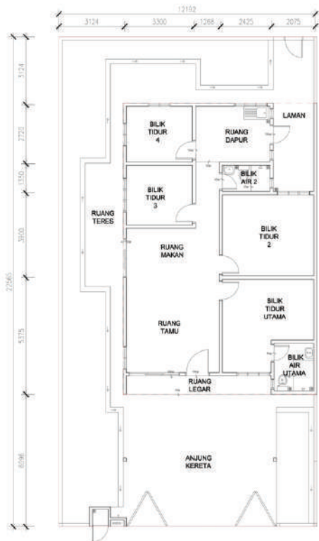
RUMAH BERKEMBAR JENIS RB1
