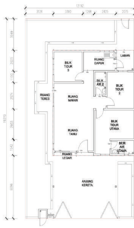
RUMAH BERKEMBAR JENIS RB2
