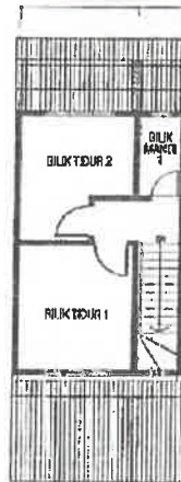
PELAN LANTAI (ARAS SATU)
