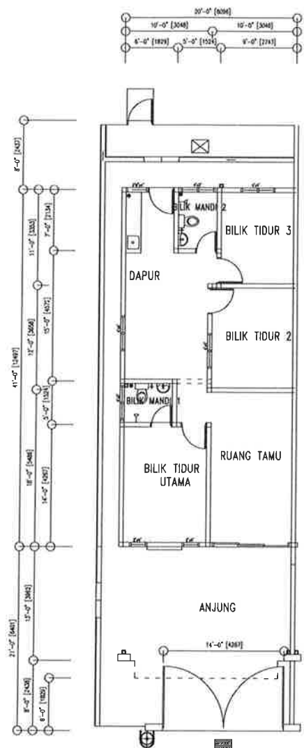
PELAN LANTAI
