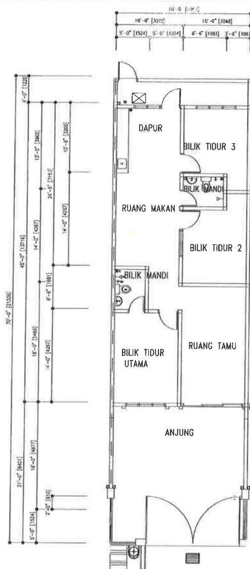
PELAN LANTAI
