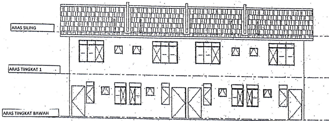
PANDANGAN BELAKANG
