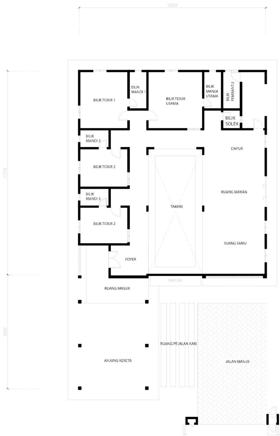
PELAN LANTAI- JENIS A
