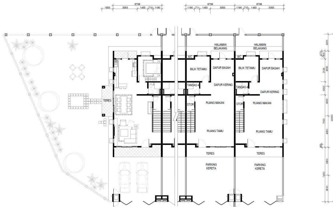
PELAN LANTAI ARAS BAWAH
