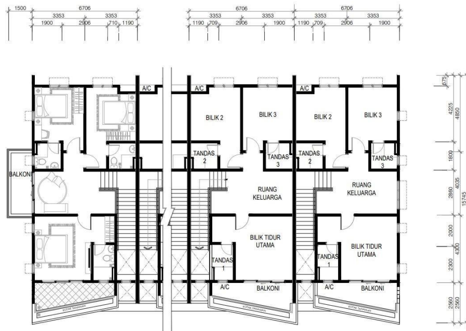
PELAN LANTAI ARAS 1
