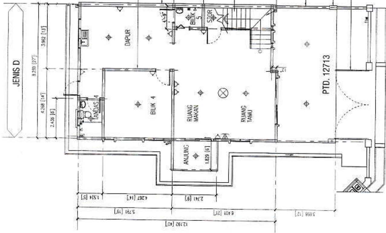
PELAN LANTAI TINGKAT BAWAH
