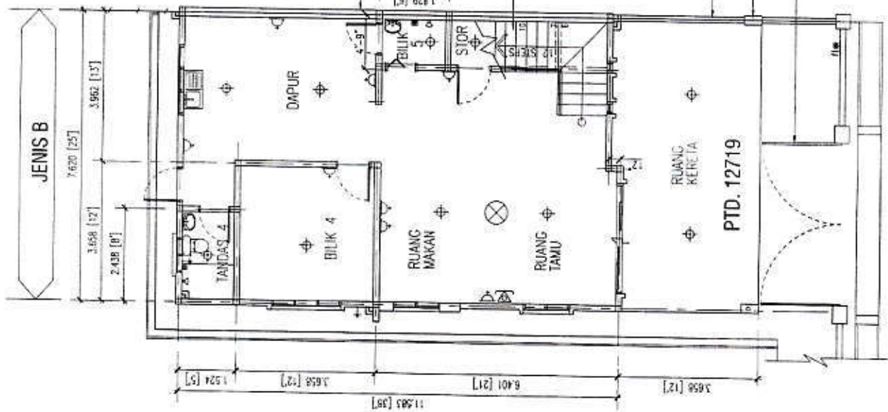
PELAN LANTAI TINGKAT BAWAH JENIS 'B' (25' X 38') RUMAH BERBANDUNG DUA TINGKAT KELUASAN LANTAI: 116.13m 2
