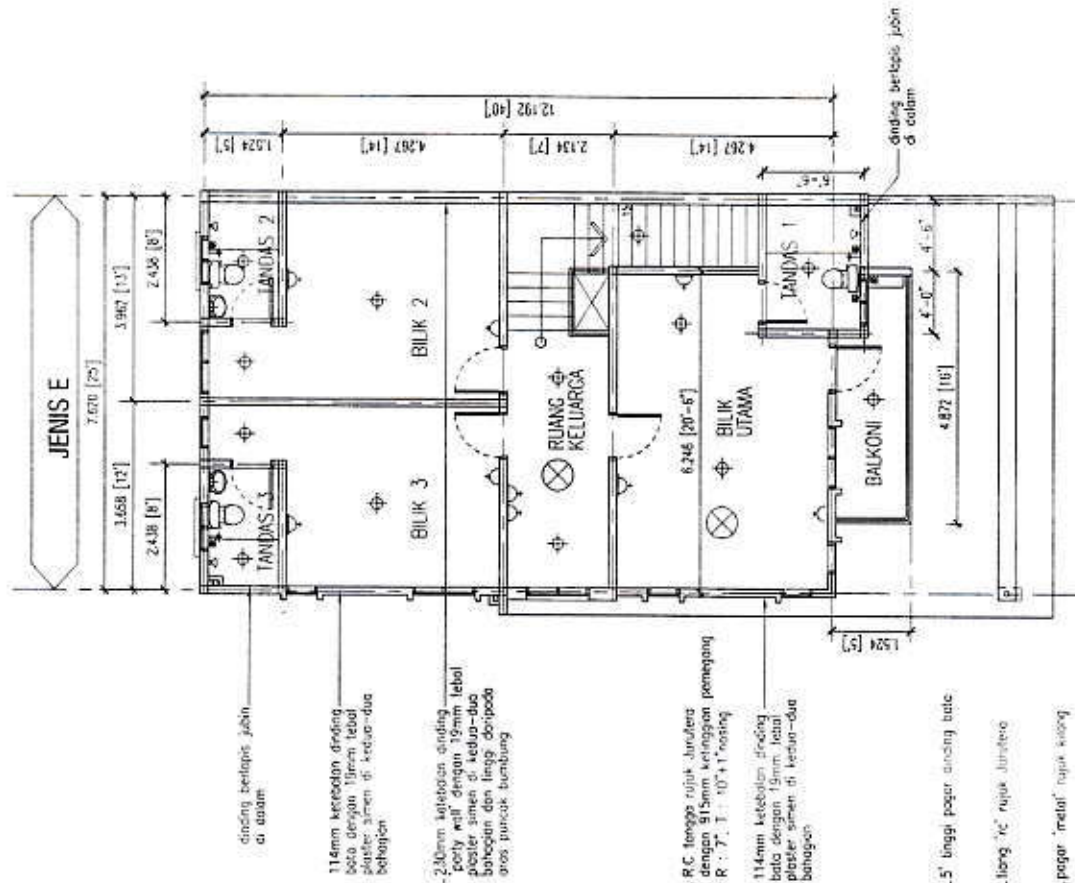
PELAN LANTAI TINGKAT SATU JENIS 'E' (25' X 40') RUMAH BERBANDUNG DUA TINGKAT KELUASAN LANTAI: 98.48m 2
