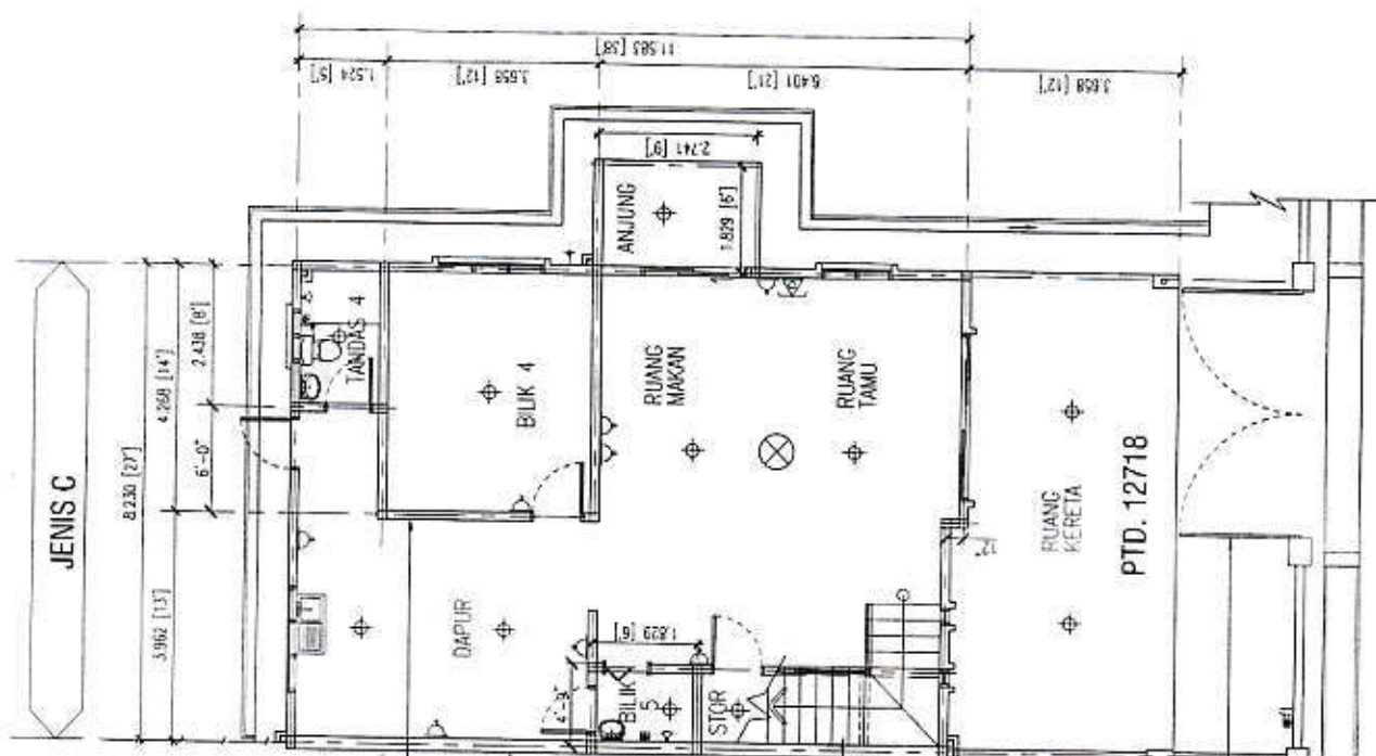
PELAN LANTAI TINGKAT BAWAH JENIS 'C' (27' X 38') RUMAH BERBANDUNG DUA TINGKAT KELUASAN LANTAI: 129.33m 2
