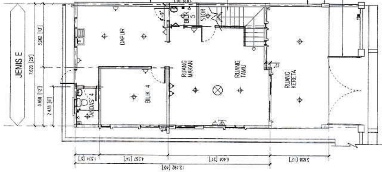
PELAN LANTAI TINGKAT BAWAH JENIS 'E' (25' X 40') RUMAH BERBANDUNG DUA TINGKAT KELUASAN LANTAI: 120.79m 2 (PTD. 12709 & PTD. 12711)
