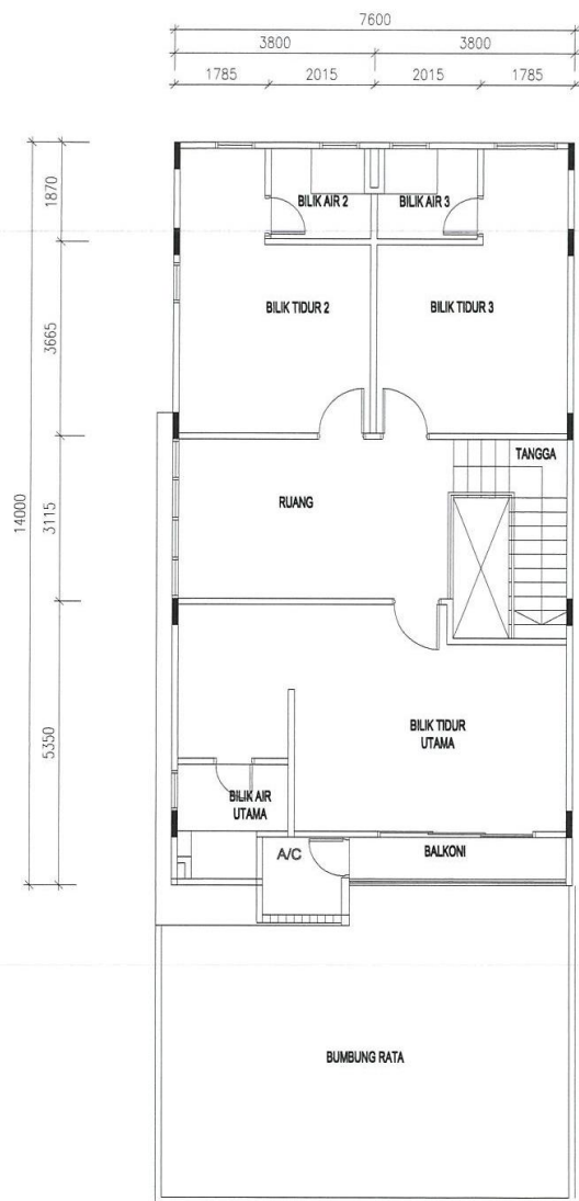
PELAN TINGKAT ATAS (JENIS C) KELUASAN BINAAN : 103.21 SQM
