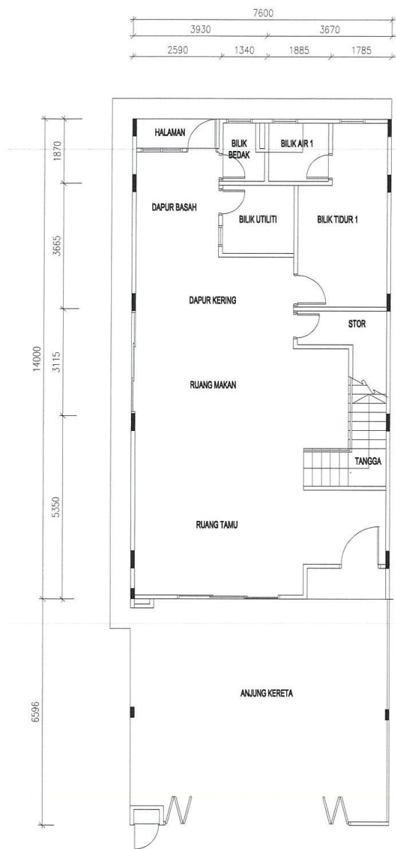
PELAN TINGKAT BAWAH (JENIS C) KELUASAN BINAAN: 115.86 SQM
