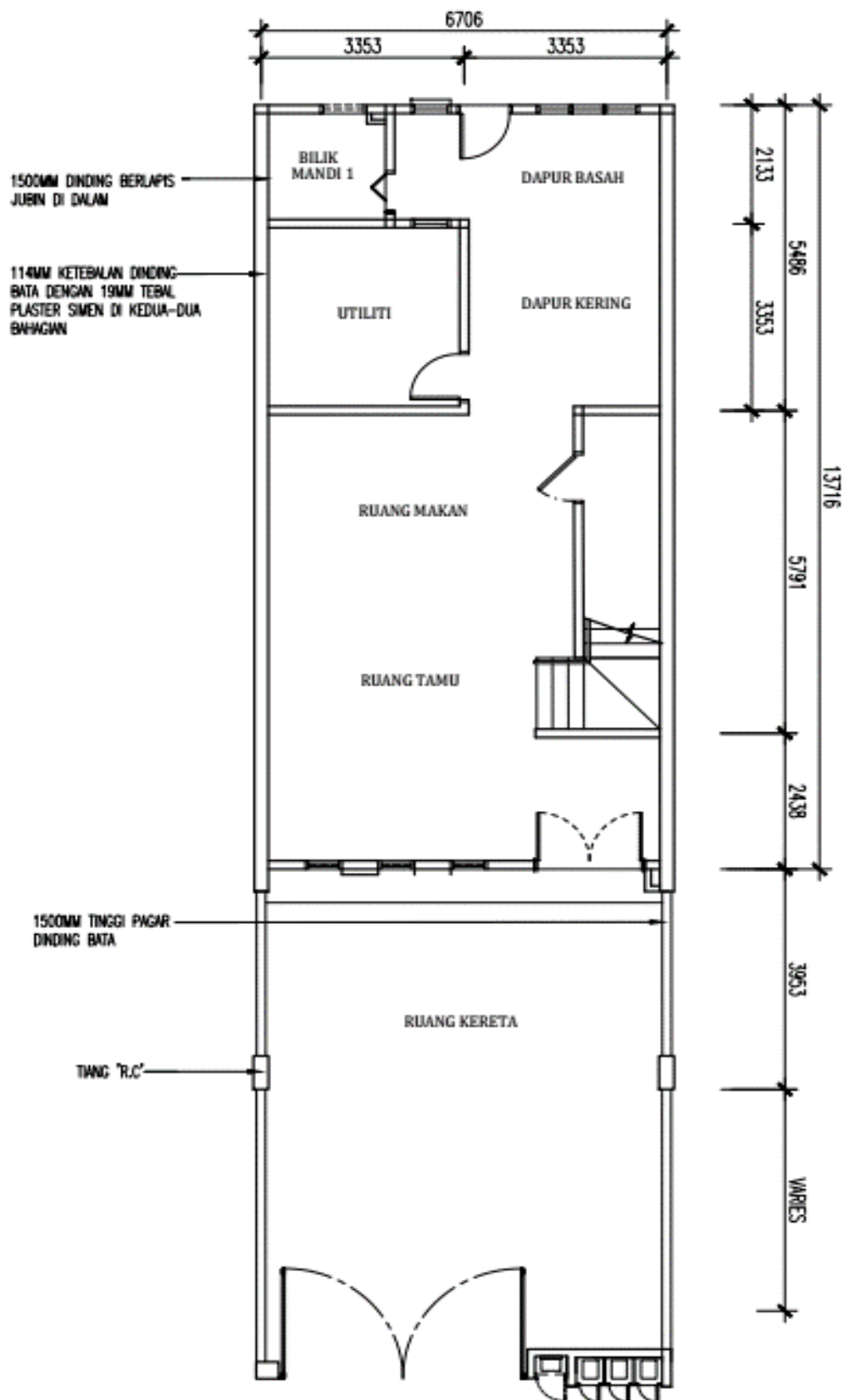
PELAN LANTAI TINGKAT BAWAH
