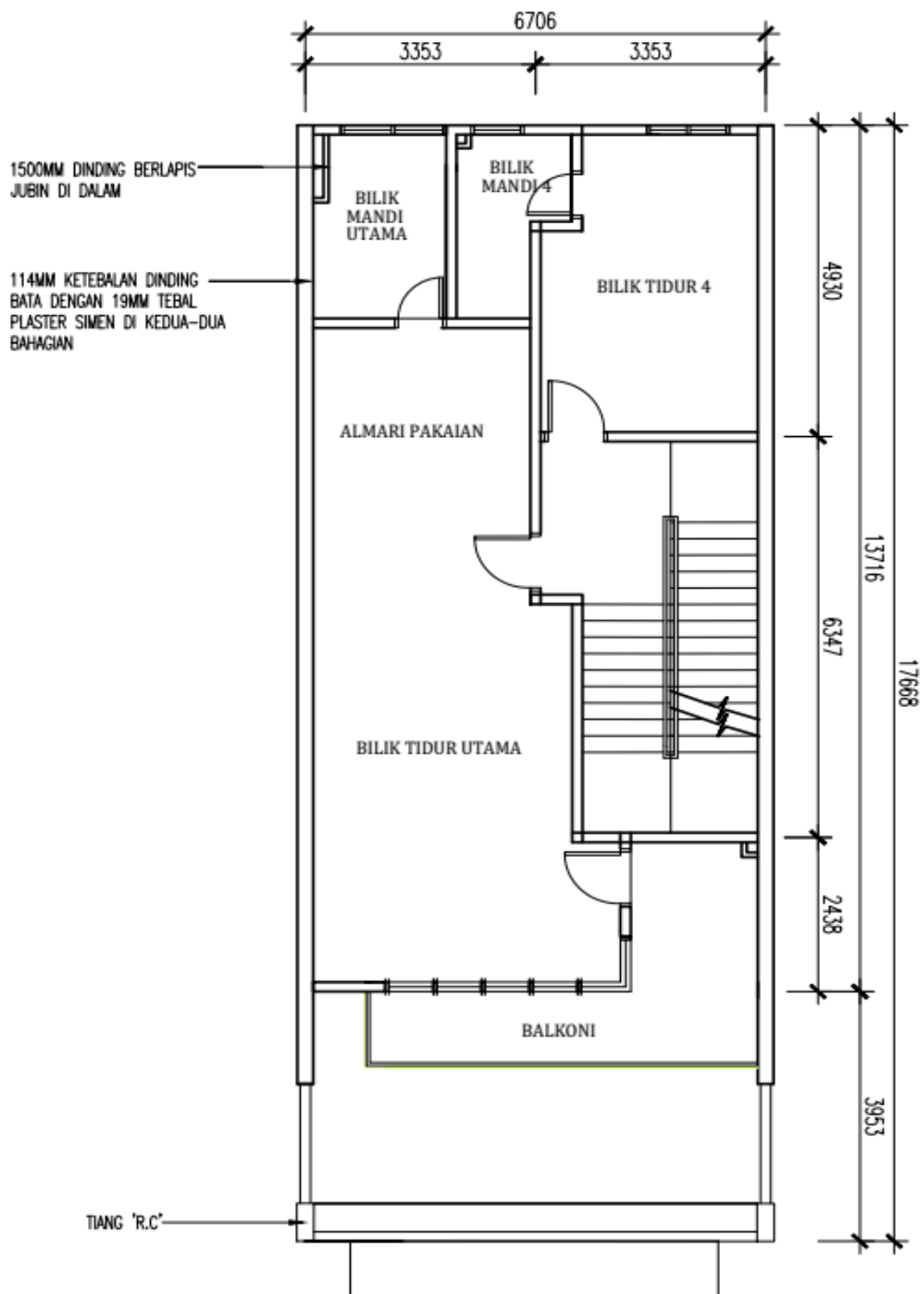
PELAN LANTAI TINGKAT KEDUA
