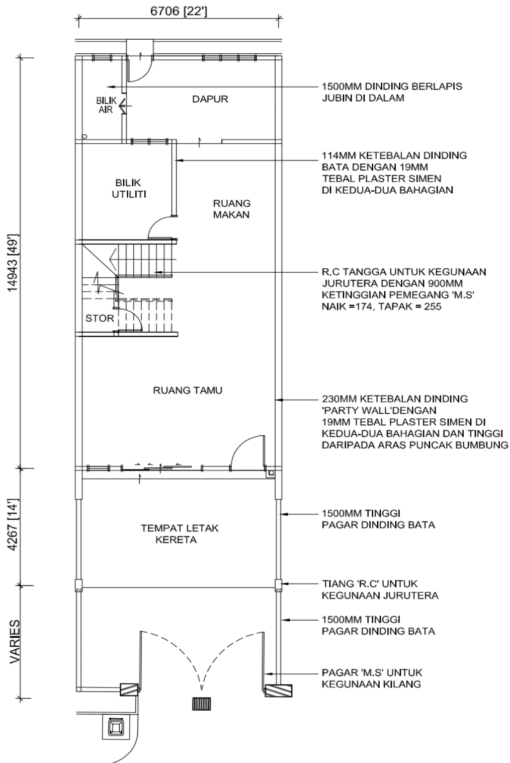
PELAN LANTAI BAWAH (LOT PERTENGAHAN)
