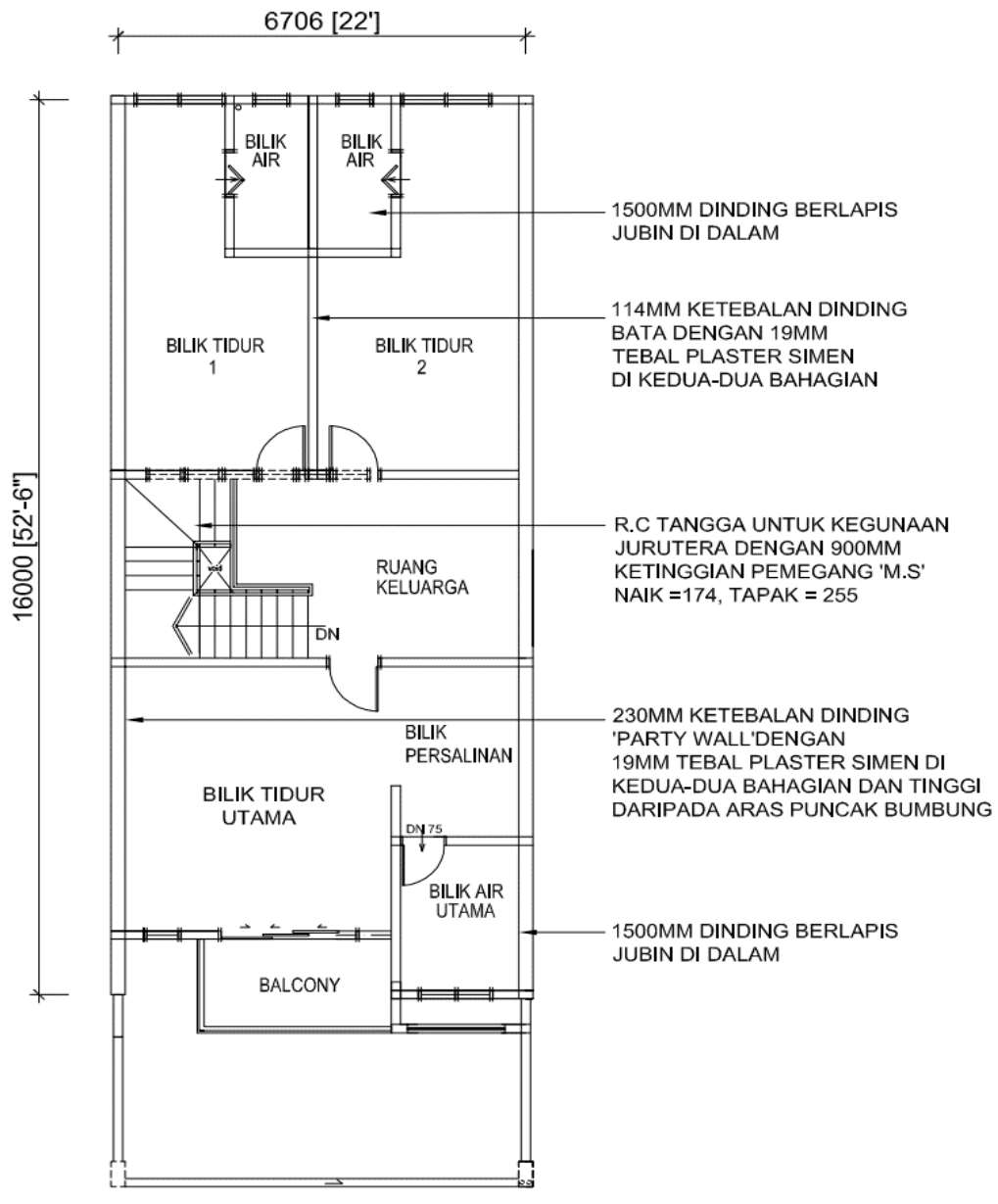
PELAN LANTAI TINGKAT SATU (LOT PERTENGAHAN)
