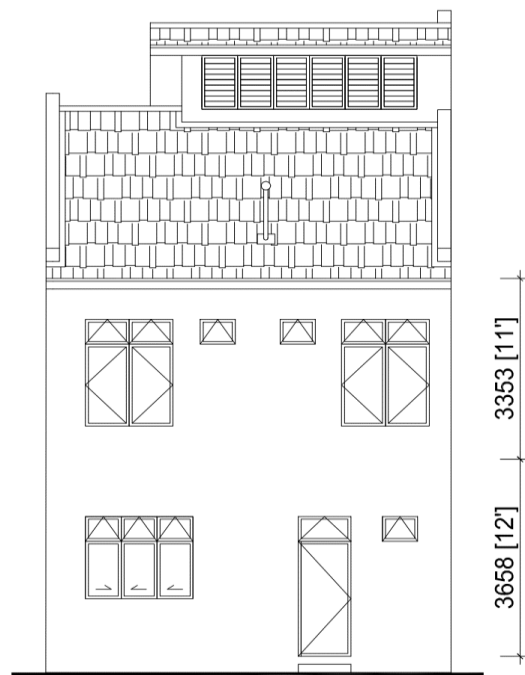
PANDANGAN BELAKANG (LOT PERTENGAHAN)
