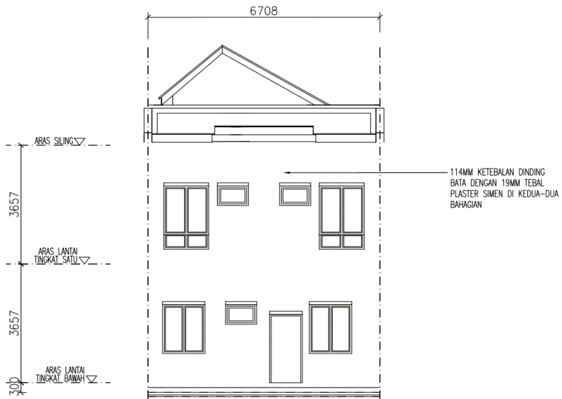
PANDANGAN BELAKANG
