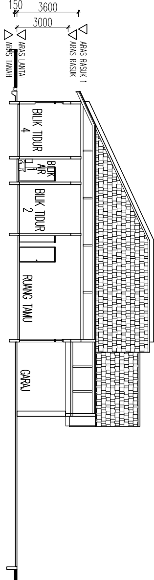
KERATAN 1
