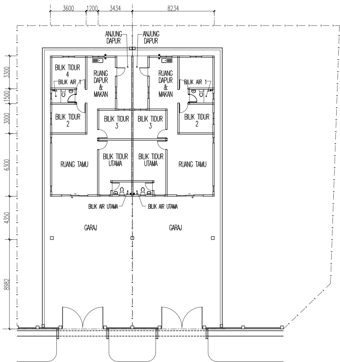
PELAN LANTAI
