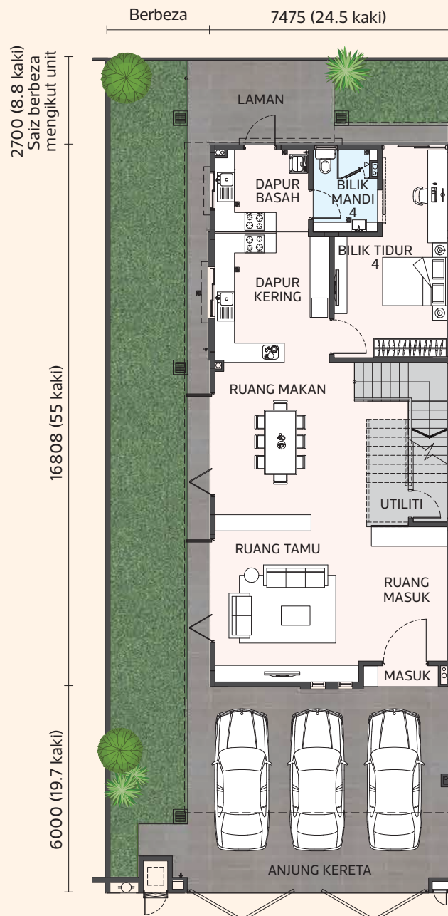
Pelan Lantai Aras Bawah
