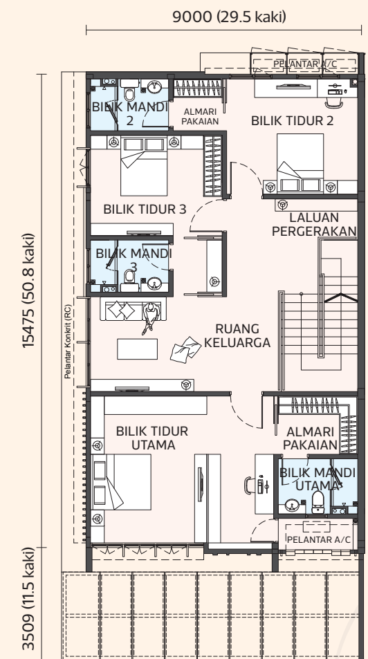
Pelan Lantai Aras Satu
