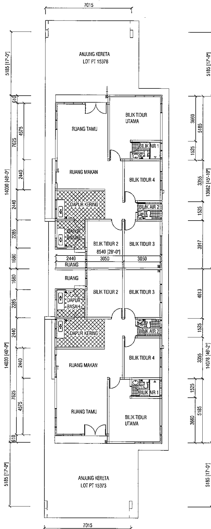
PELAN LANTAI RUMAH BERKEMBAR SETINGKAT (TYPE B)
