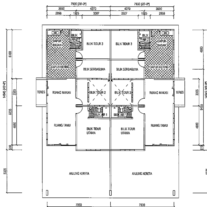
PELAN LANTAI RUMAH BERKEMBAR SETINGKAT (TYPE A)
