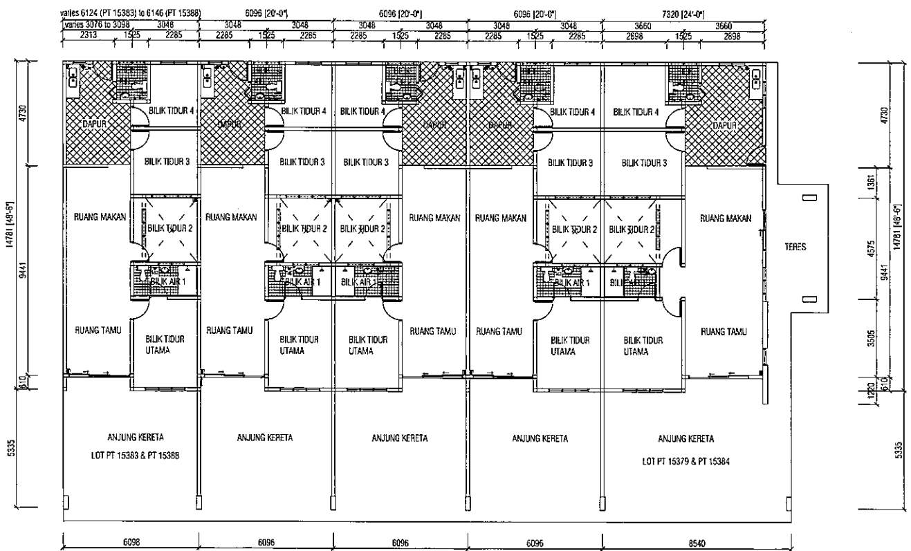
PELAN LANTAI RUMAH TERES SETINGKAT
