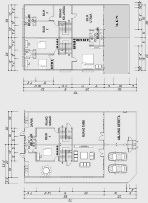
TINGKAT BAWAH
