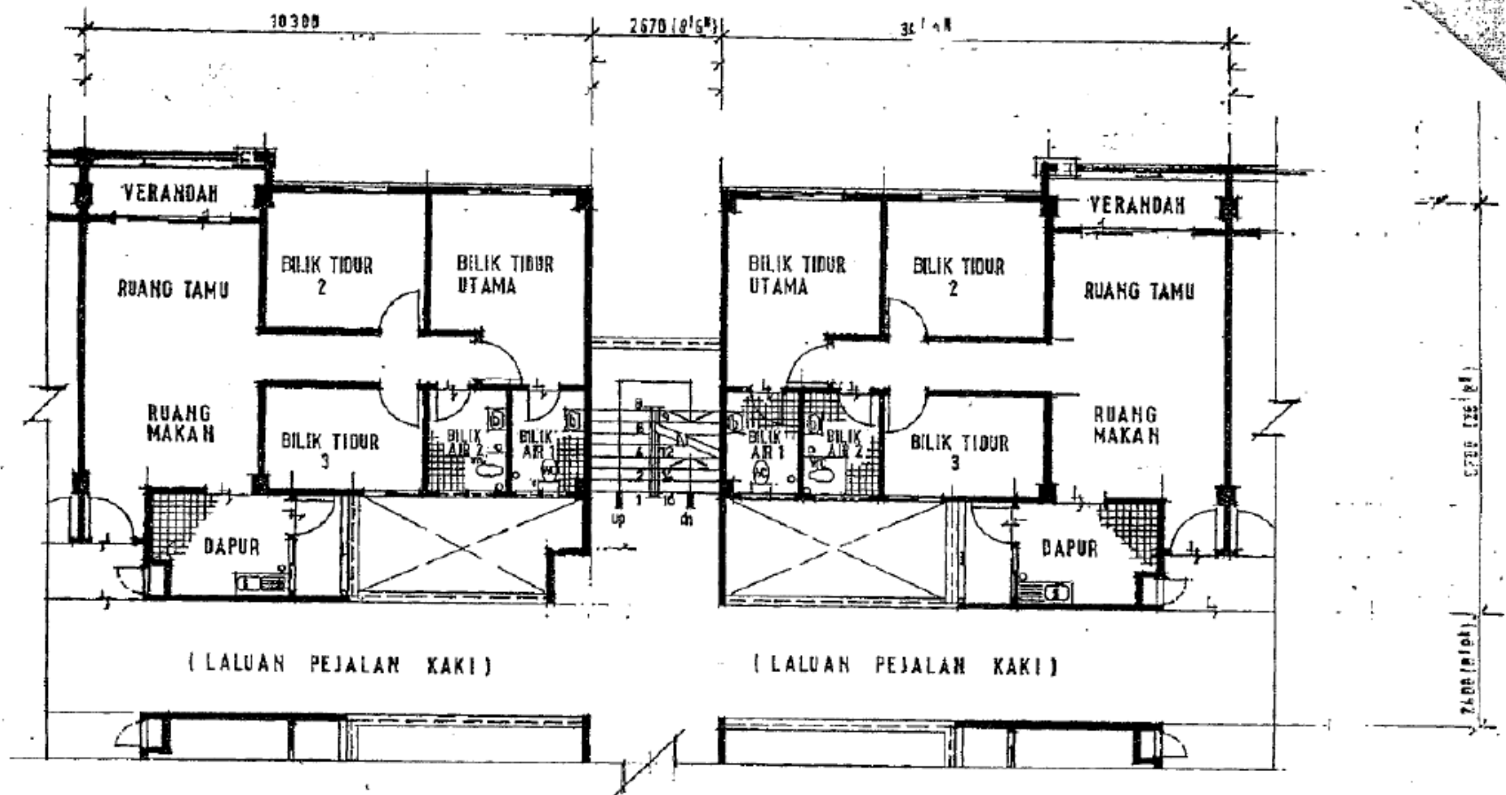
PELAN TINGKAT 1 HINGGA TINGKAT 6 (RUMAH PANGSA KOS SEDERHANA RENDAH 7 TINGKAT)
